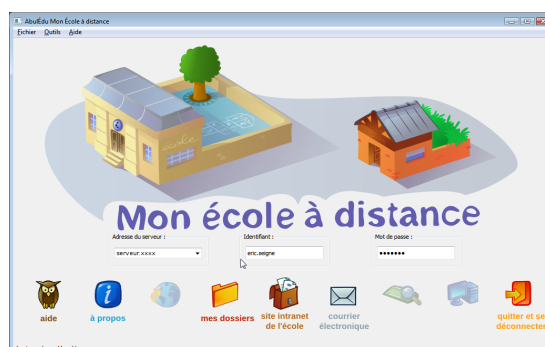
Illustration 2: Connexion établie
